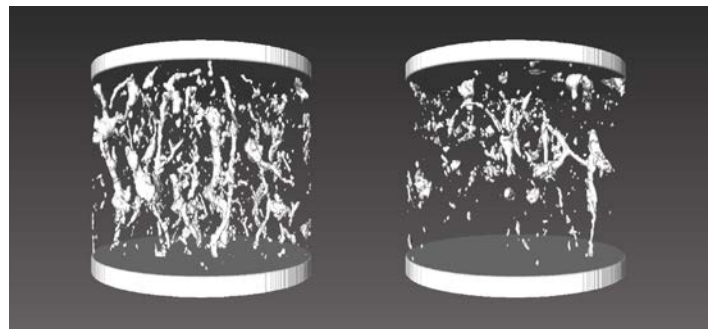
Fig. 5.3. CT scan macro poriën van de bodem (kleigrond) van ongestoorde bodem (links) en (29 jaar geleden) belaste bodem met 50 kN (Schjønning et al., 2015).
