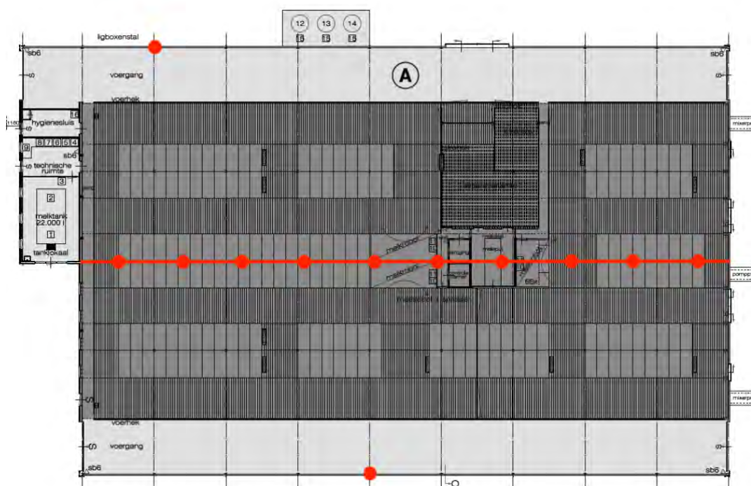
Figuur B2.2 Staluiterslijk en -indeling, inclusief oriëntatie van de stal en positie meetapparatuur (sample line en 2 buitenmeetpunten).
