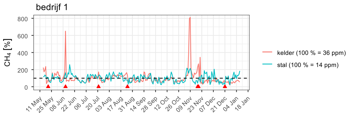
Figuur 10A: Relatieve methaanconcentraties in de kelder (rode lijn) en stal (groene lijn), met mixmomenten (rode driehoekjes) op bedrijf 1.
