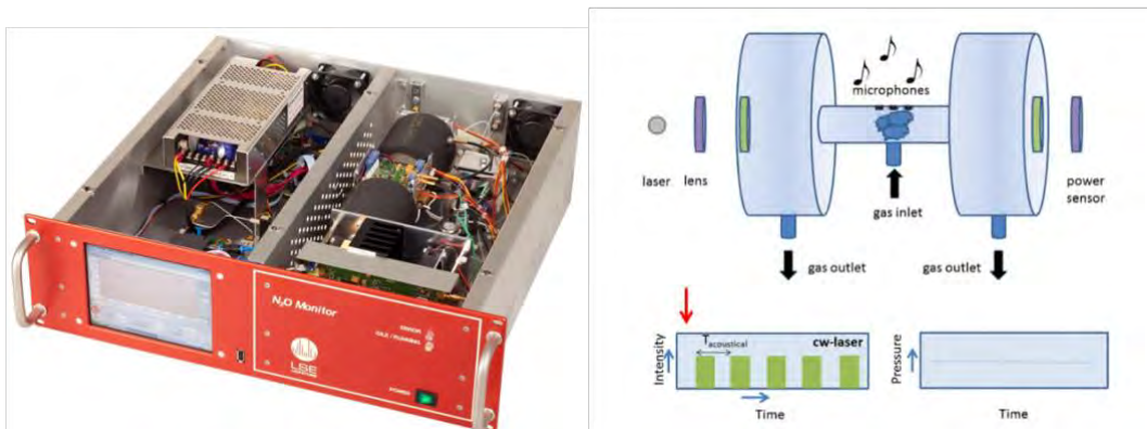
Figuur B1.3 Voor het meten van de CO 2 wordt gebruik gemaakt van infrarood (NDIR) metingen.
